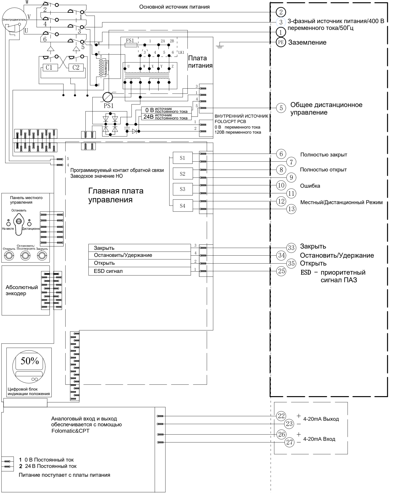
Электрическая схема №1-400-24-4-N-1 Серия VAD
