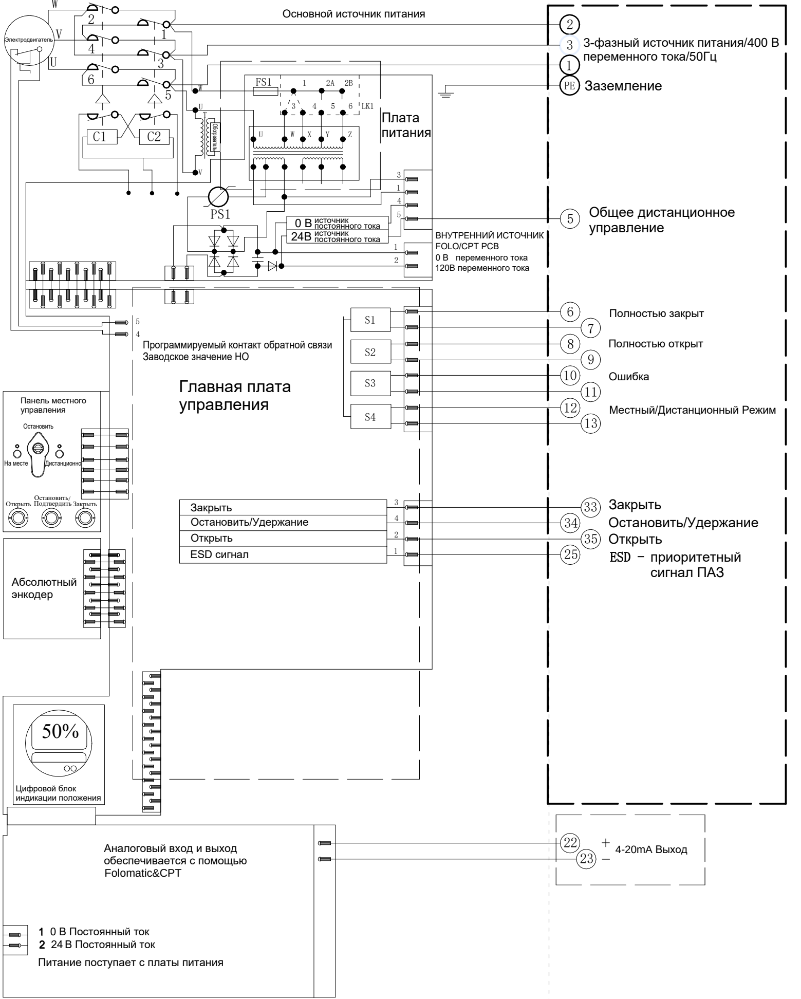
Электрическая схема №1-400-24-4-N-3 Серия VAD
