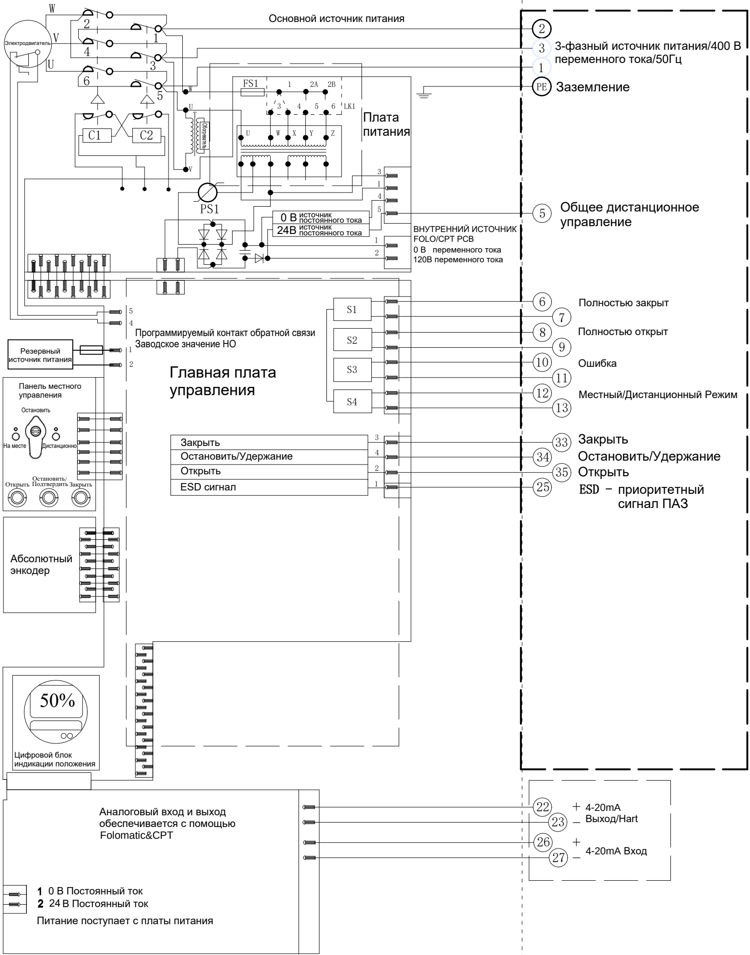
Электрическая схема №1-400В-24-4-HR-1 Серия VAD
