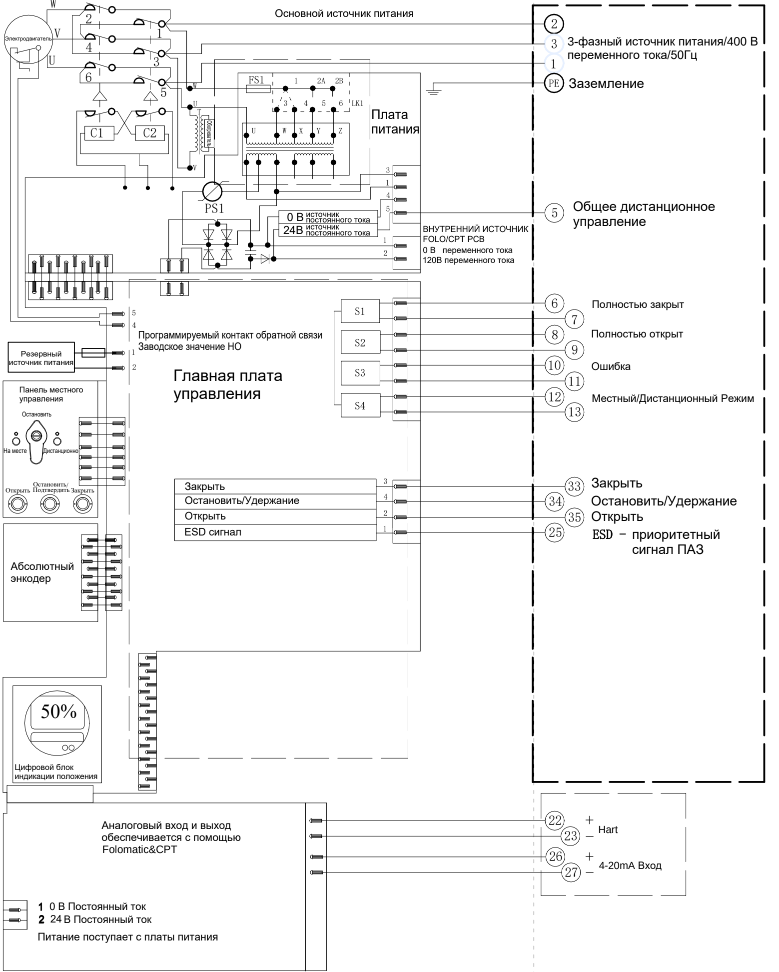
Электрическая схема №1-400B-24-4-HR-2 Серия VAD
