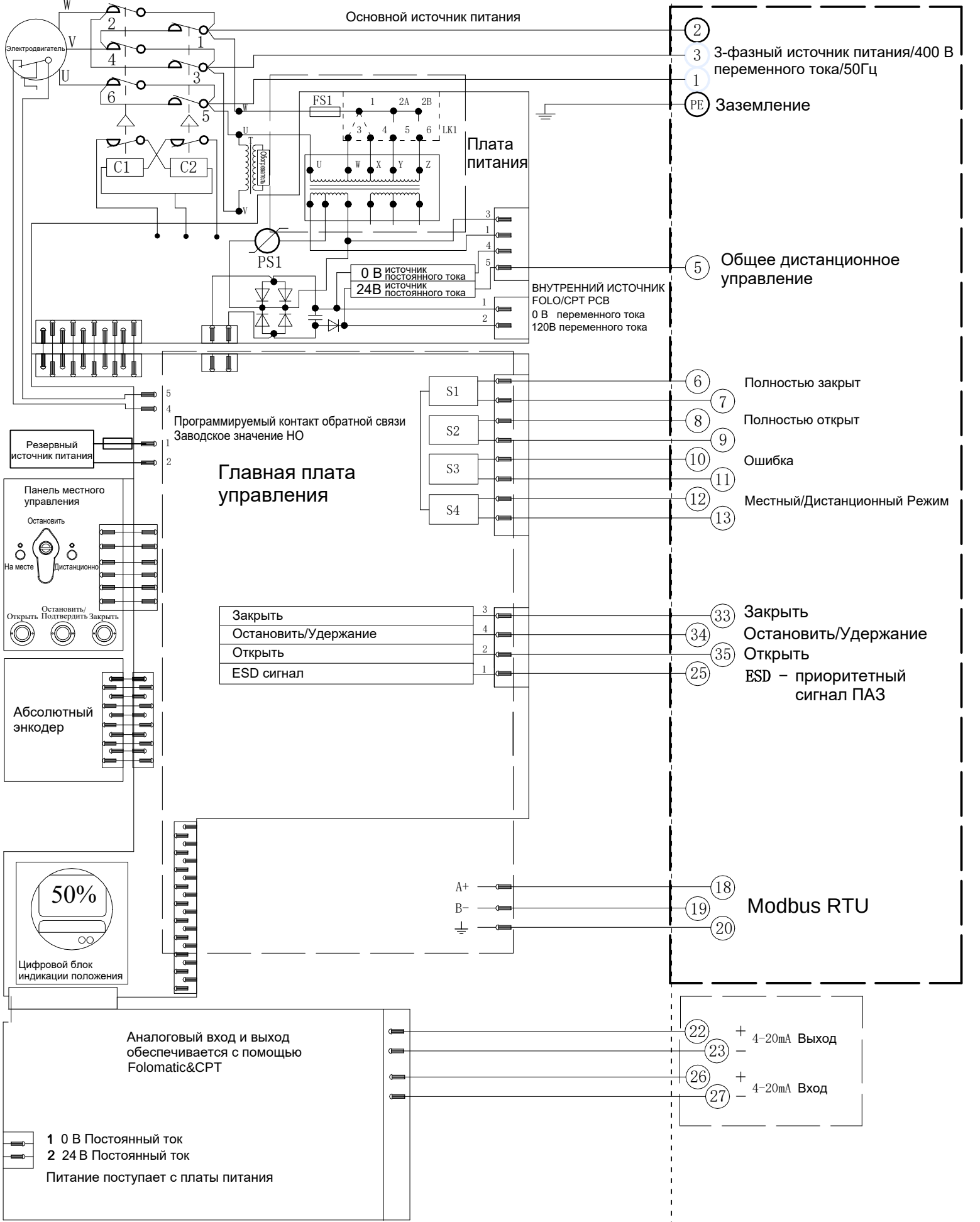
Электрическая схема №1-400B-24-4-MR-1 Серия VAD
