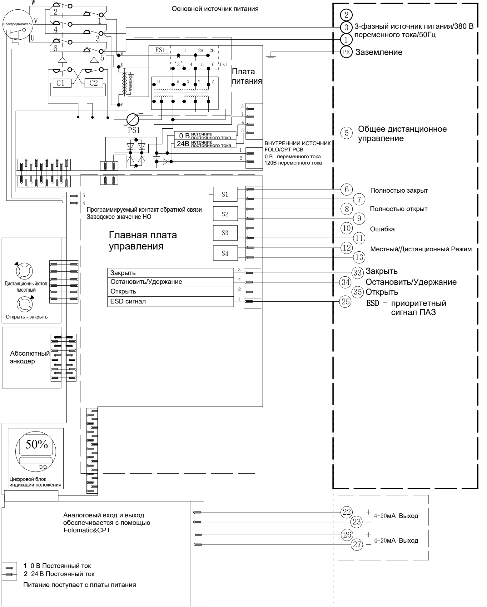
Электрическая схема №1-380-24-4-N-8 Серия VAD
