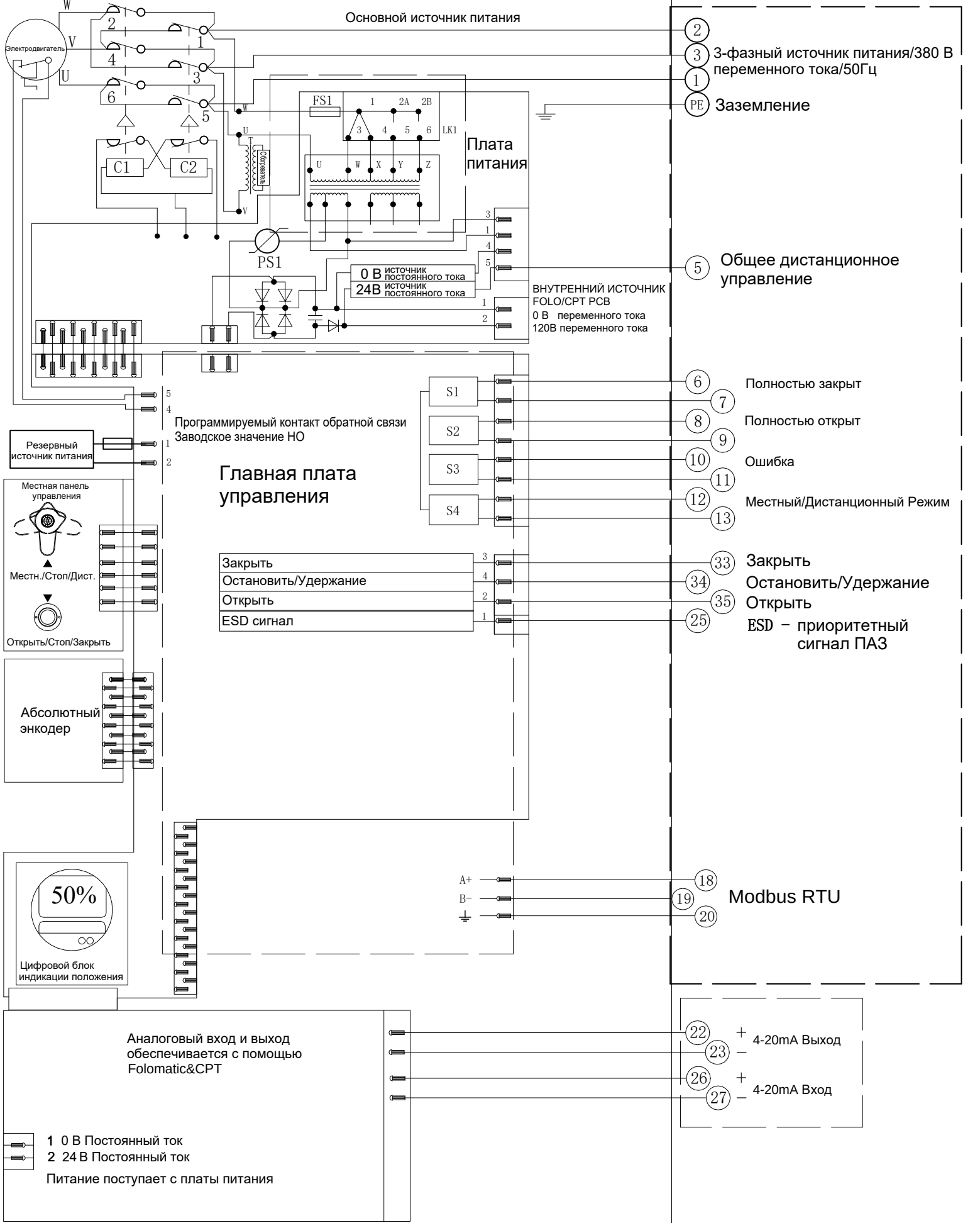
Электрическая схема №1-380В-24-4-MR-1 Серия VAD
