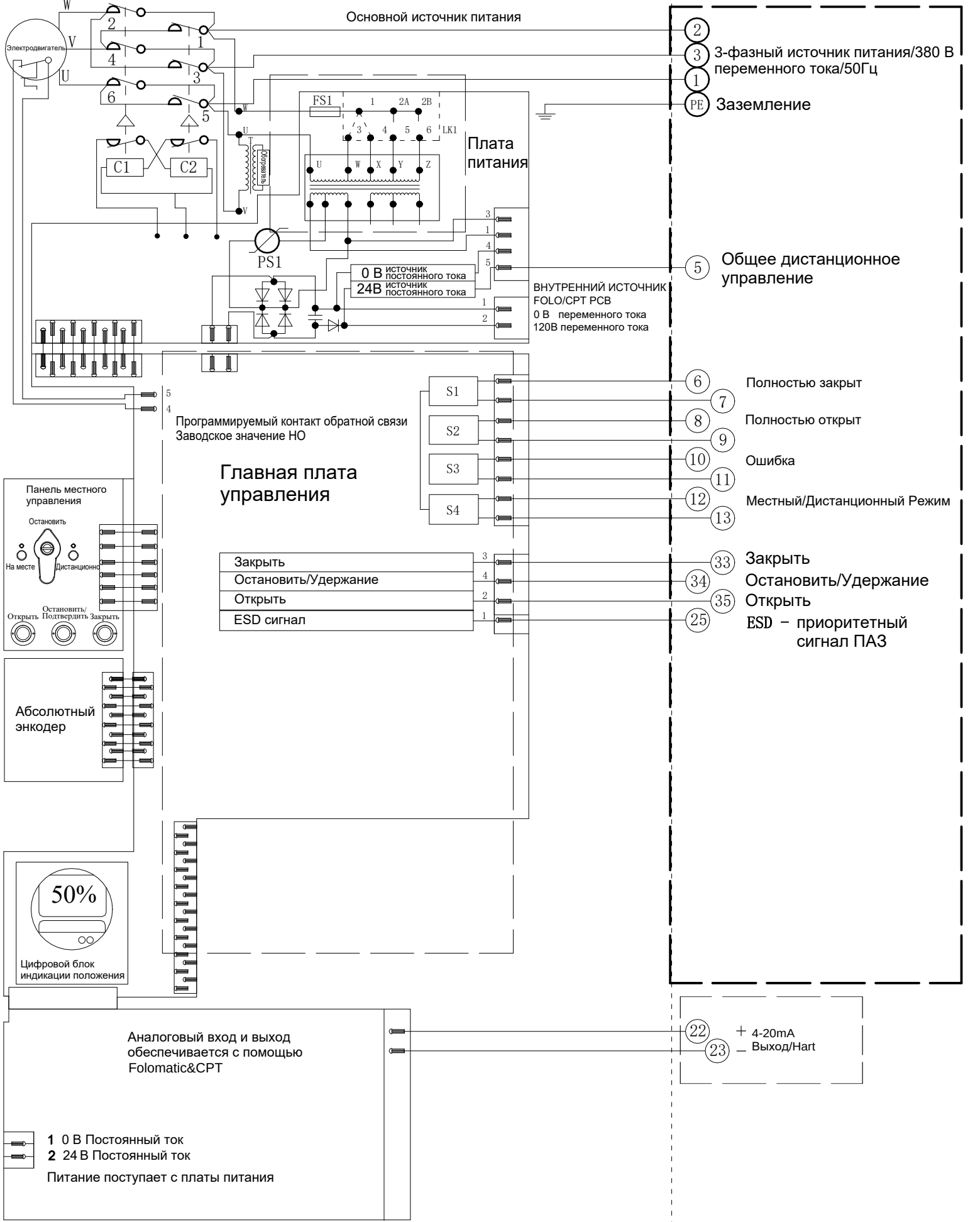
Электрическая схема №1-380-24-4-HR-3 Серия VAD
