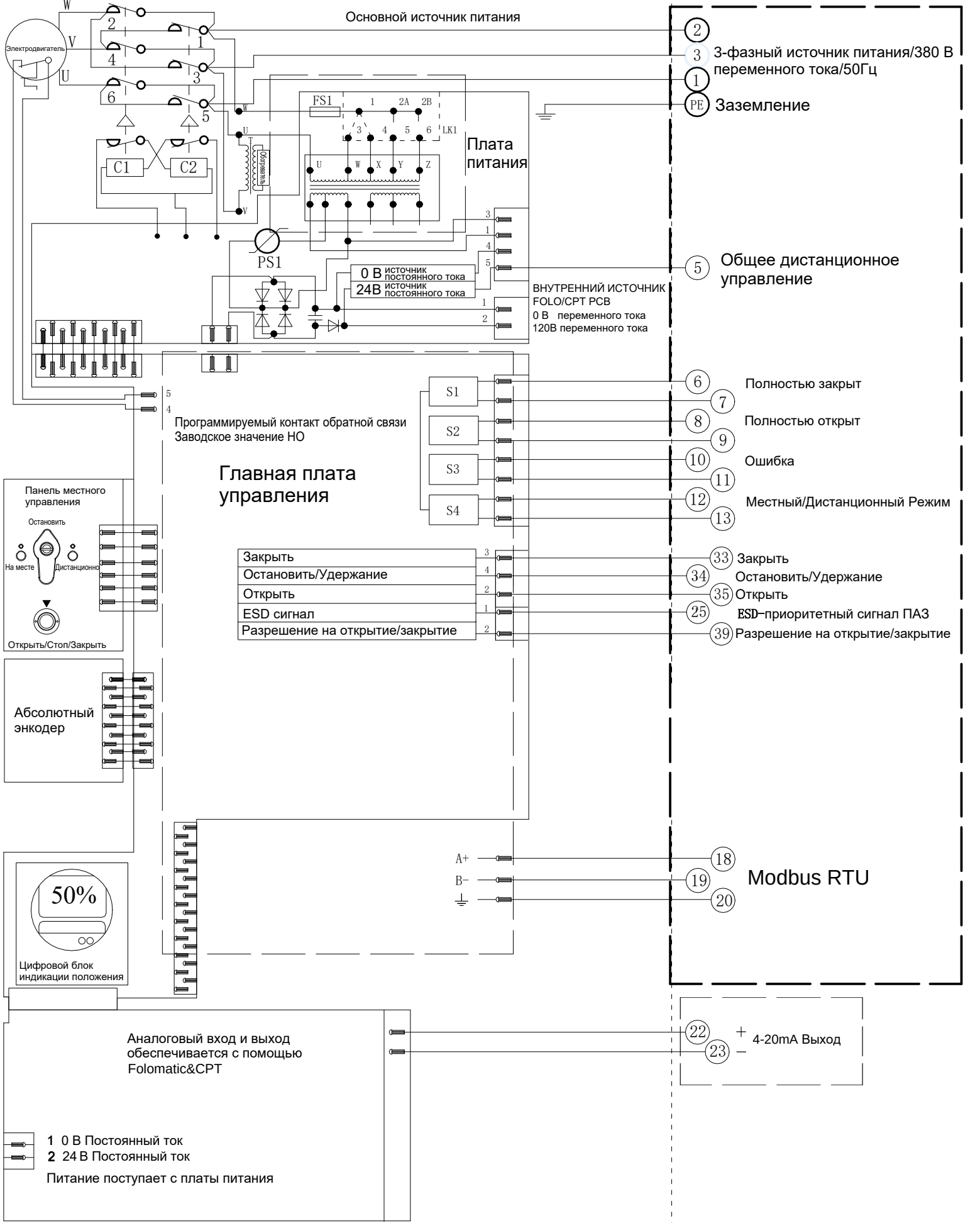
Электрическая схема №1-380-24-4-MR-3 Серия VAD
