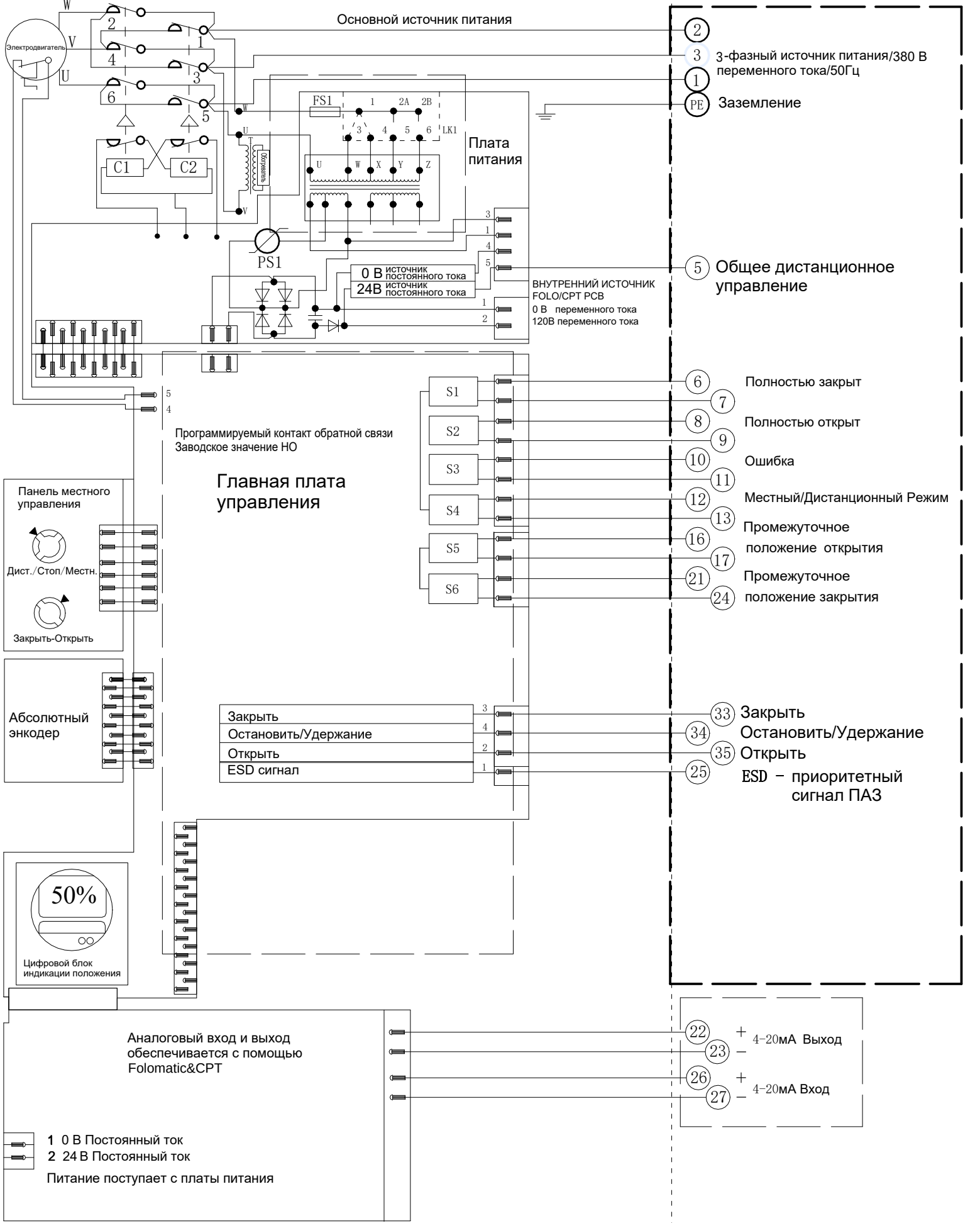
Электрическая схема № 1-380-24-6-N-1 Серия VAD
