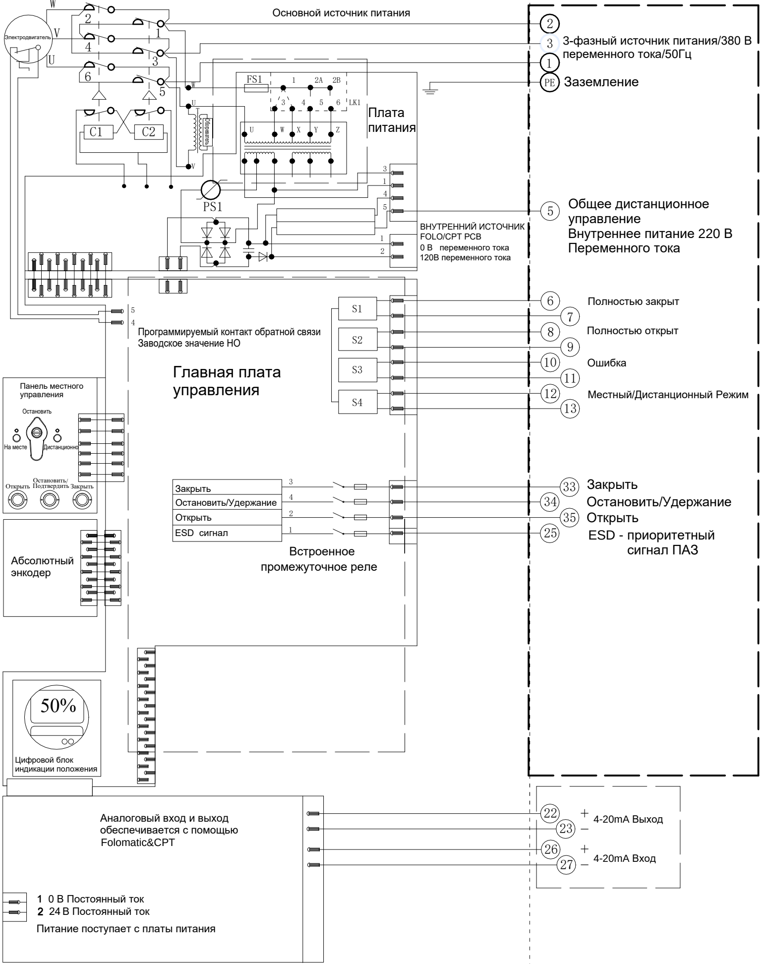
Электрическая схема №1-380-220-4-N-1 Серия VAD
