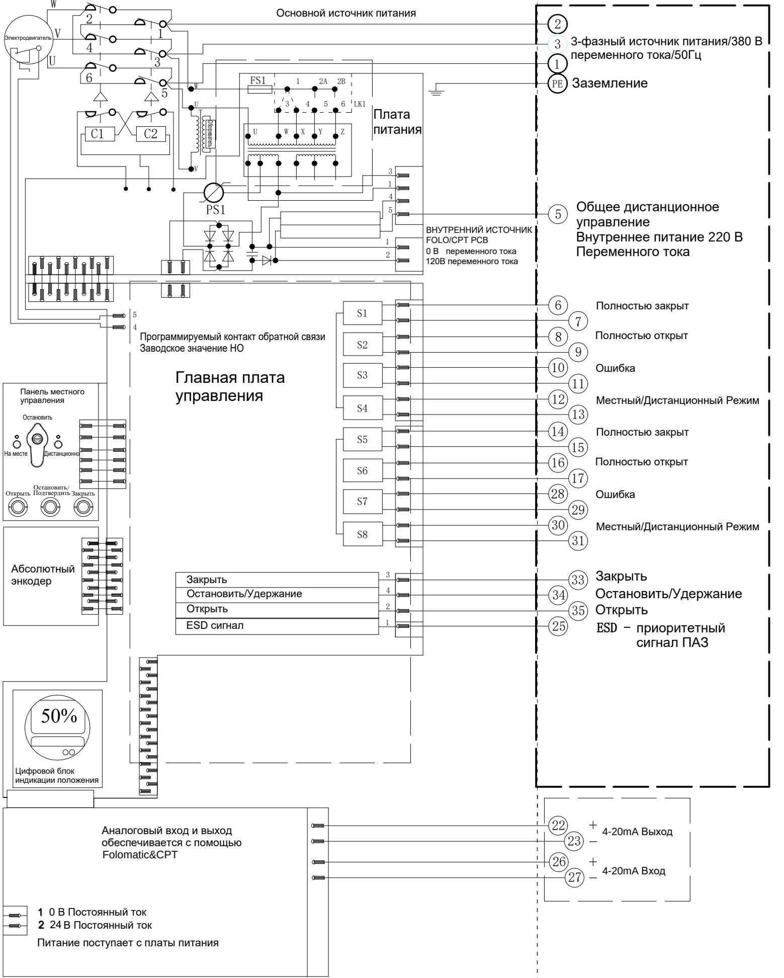
Электрическая схема №1-380-220-8-N-1 Серия VAD
