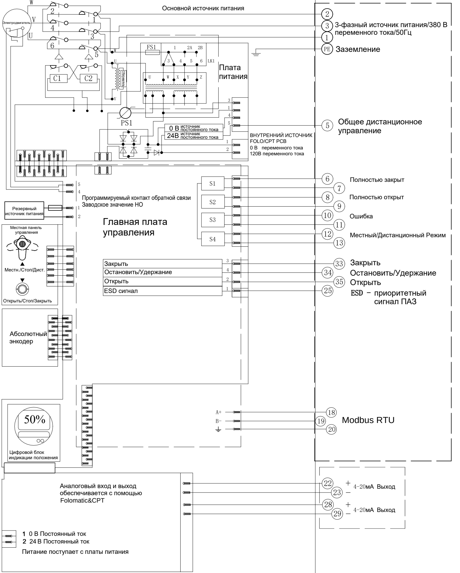
Электрическая схема №1-380В-24-4-MR-8 Серия VAD
