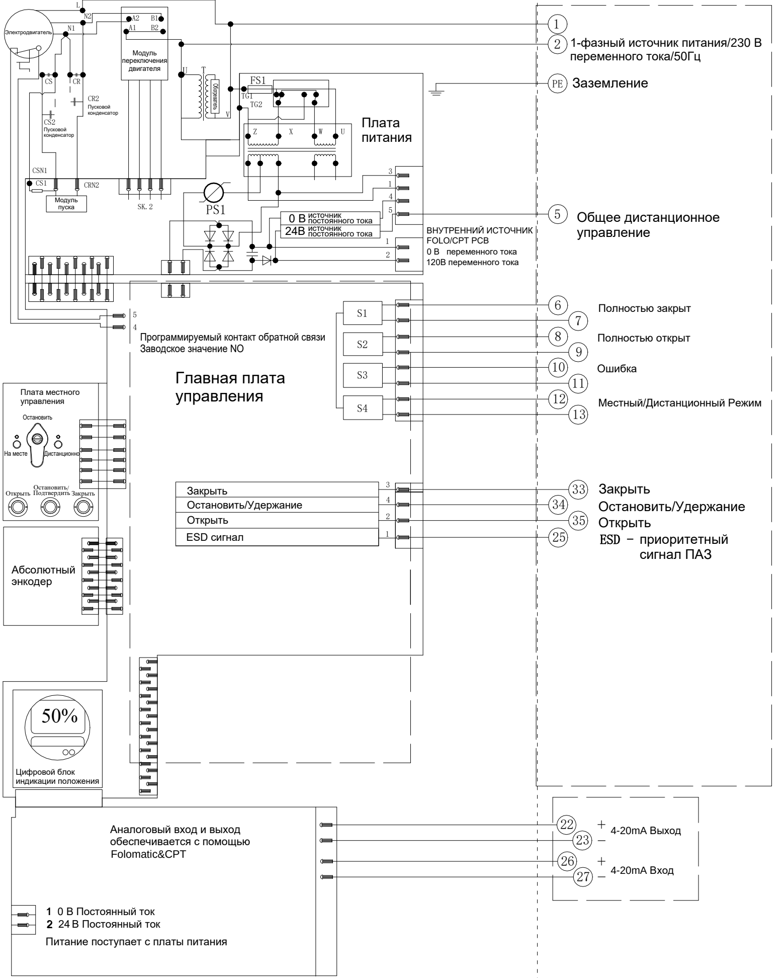
Электрическая схема №1-230-24-4-N-1 Серии VAD
