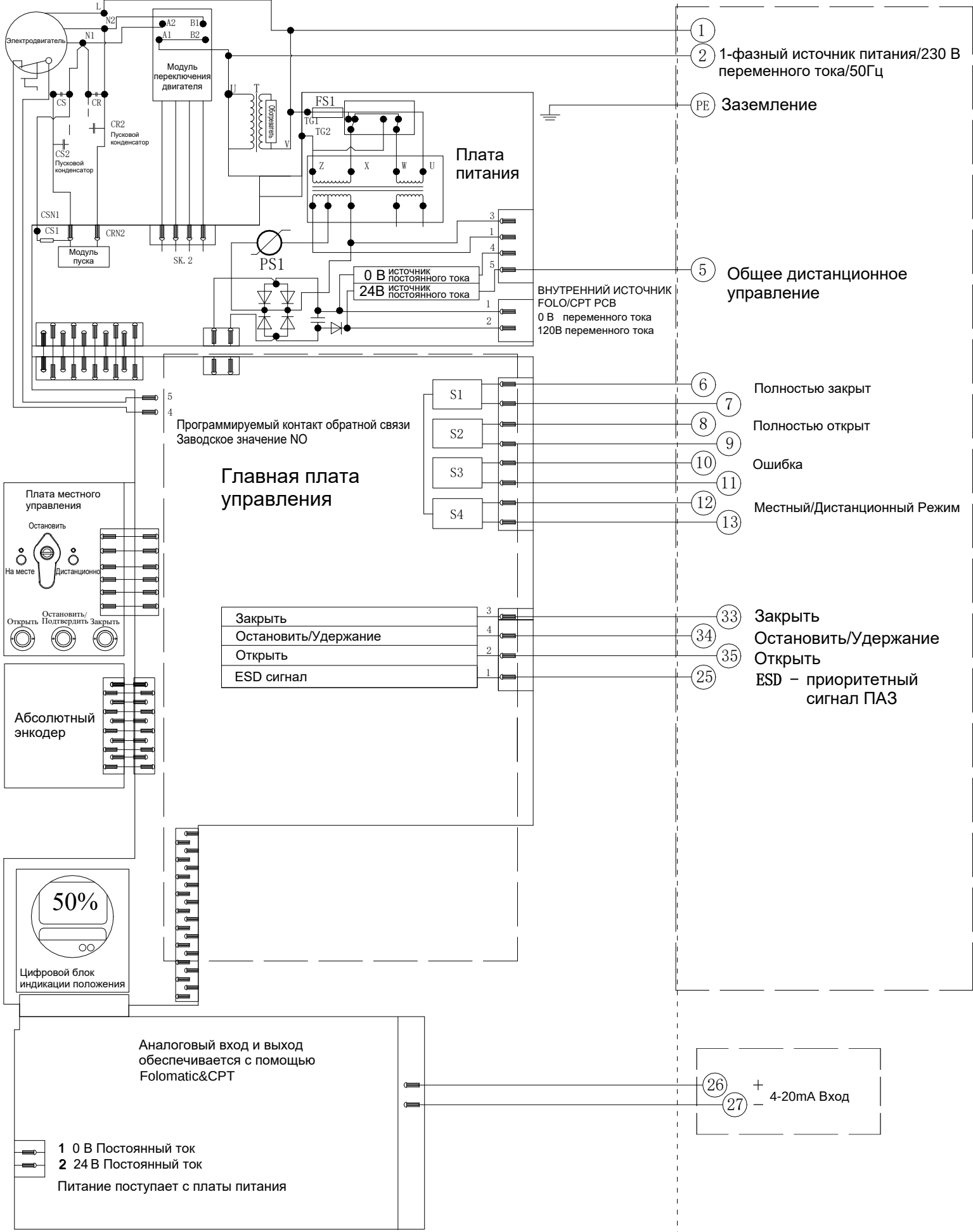
Электрическая схема №1-230-24-4-N-2 Серии VAD
