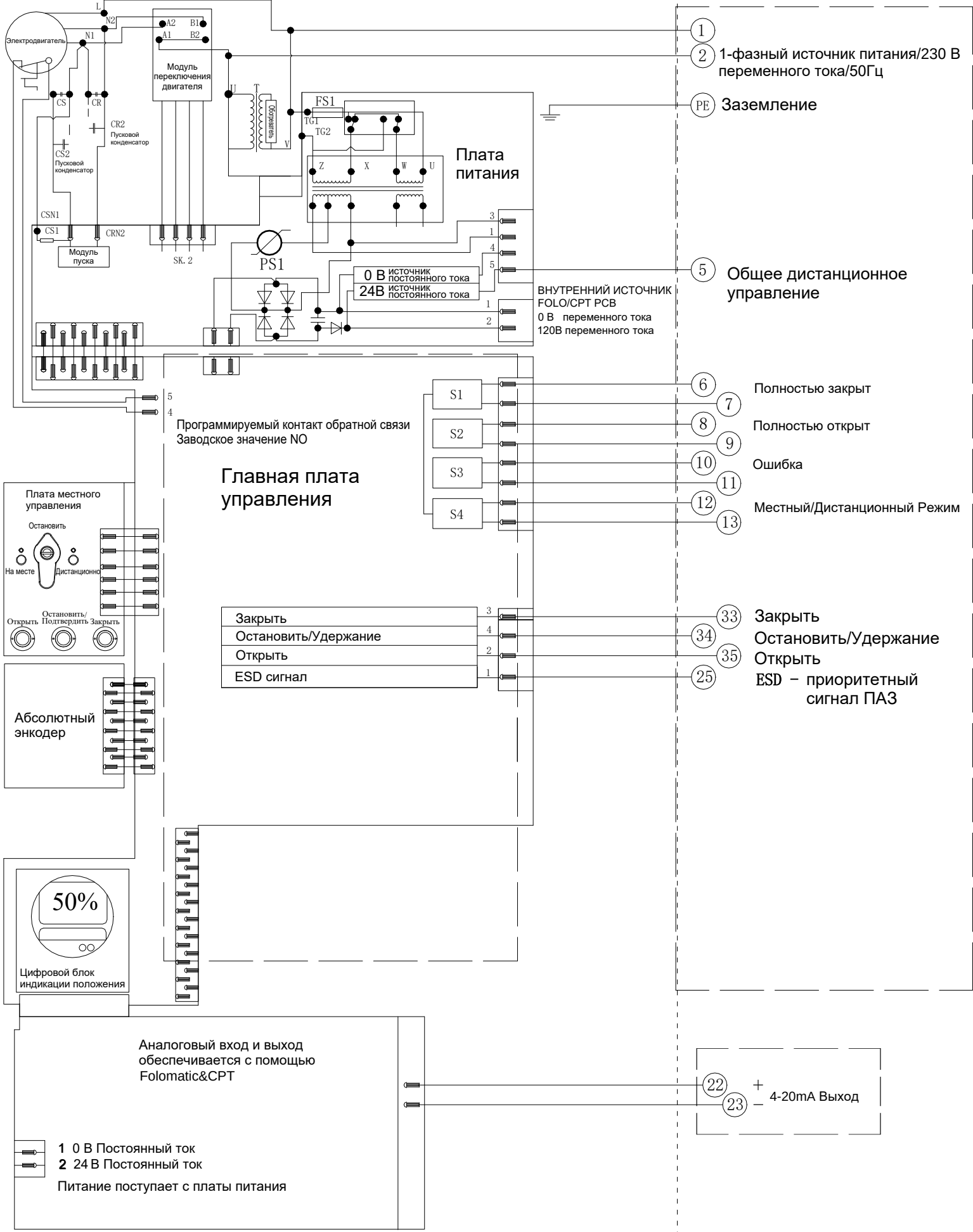
Электрическая схема №1-230-24-4-N-3 Серии VAD
