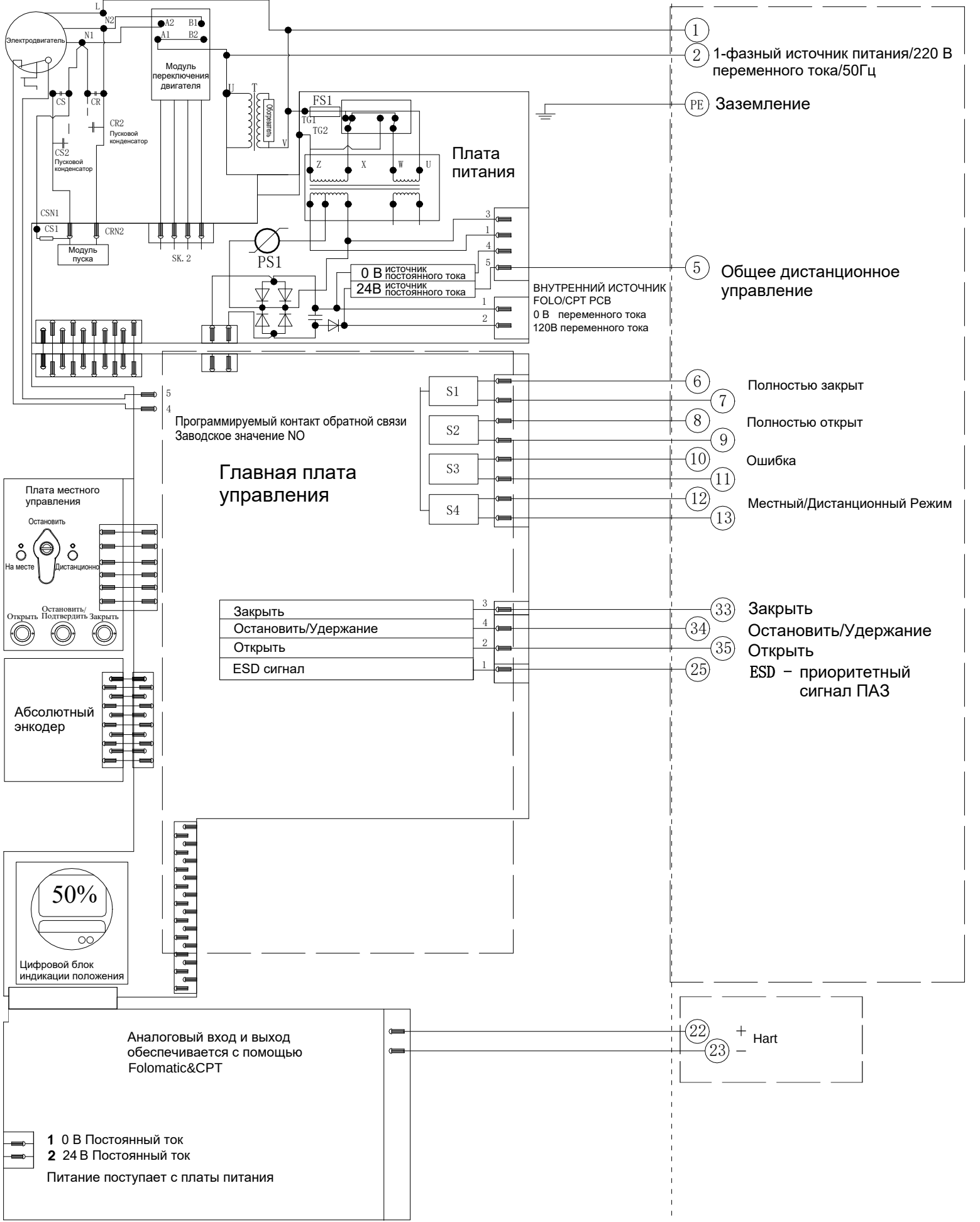
Электрическая схема №1-220-24-4-HR-0 Серия VAD
