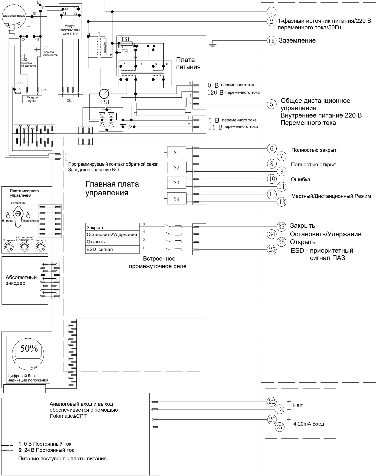
Электрическая схема №1-220-220-4-HR- 2 Серия VAD
