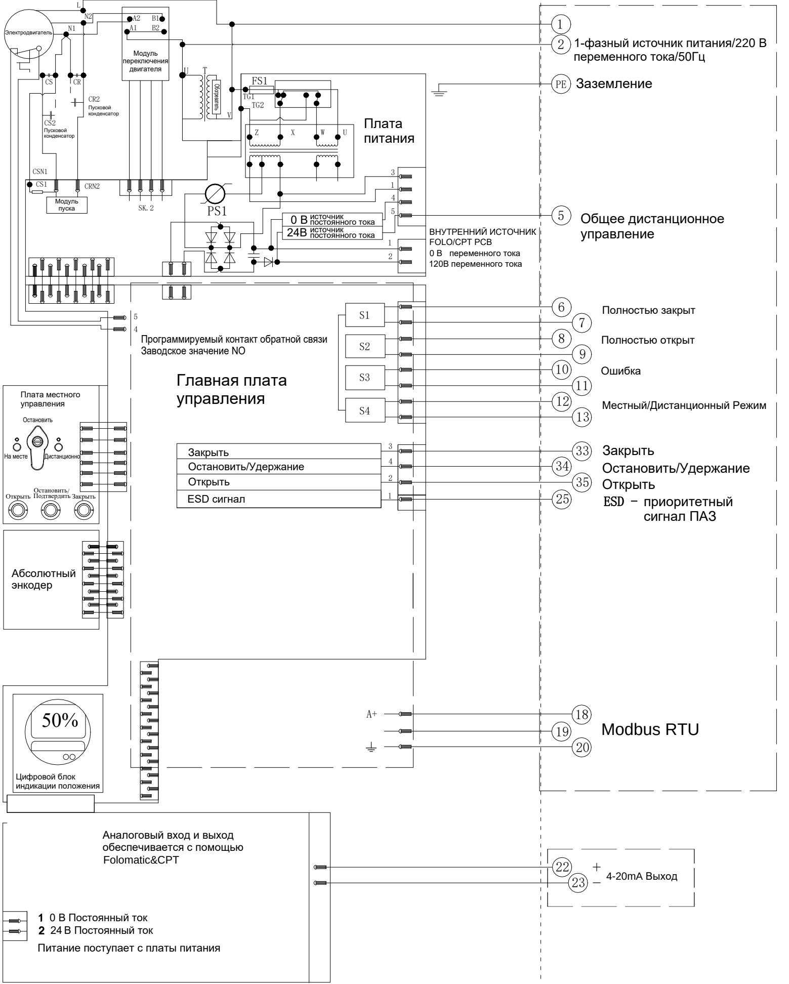
Электрическая схема №1-220-24-4-MR-3 Серия VAD
