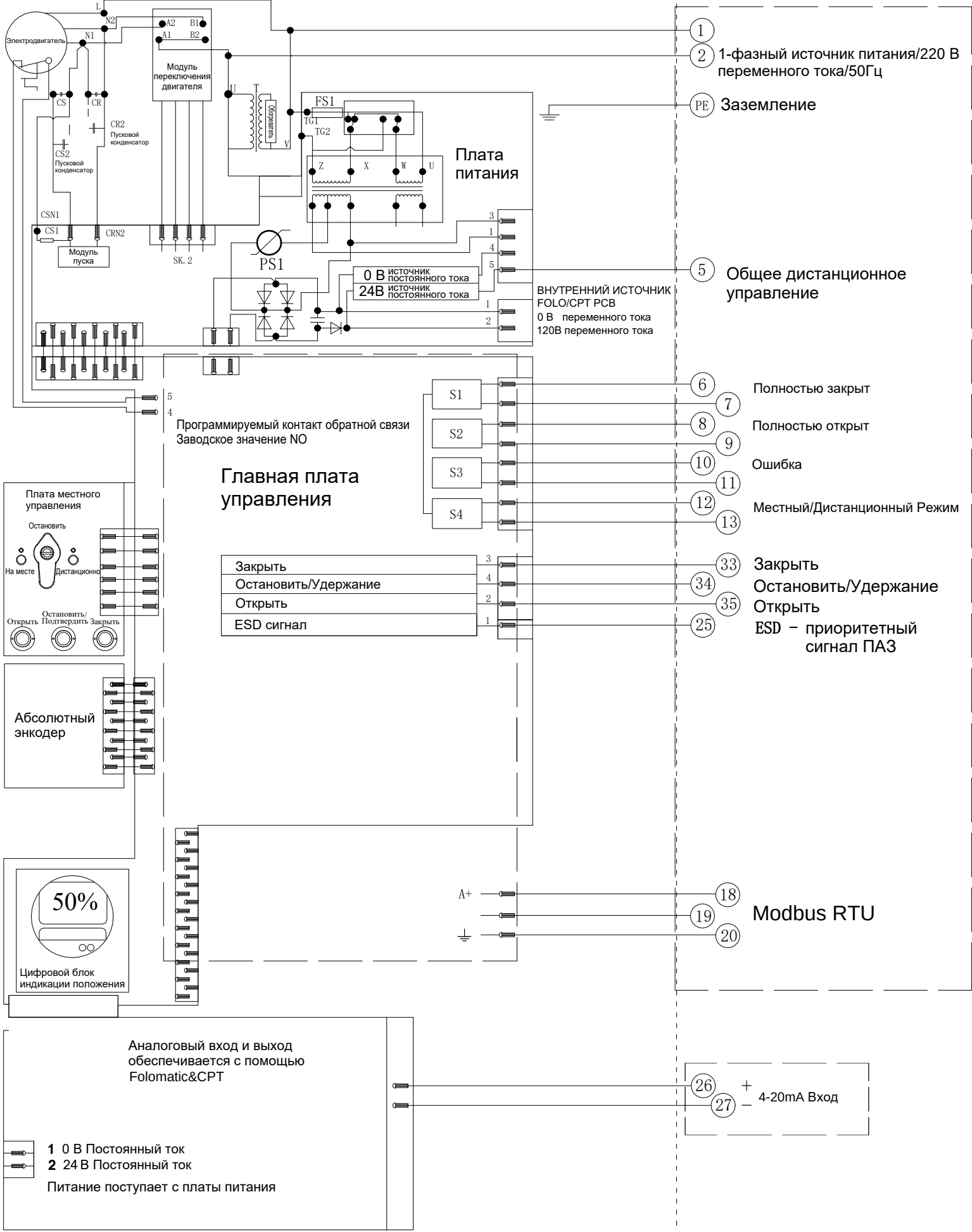
Электрическая схема №1-220-24-4-MR-2 Серия VAD
