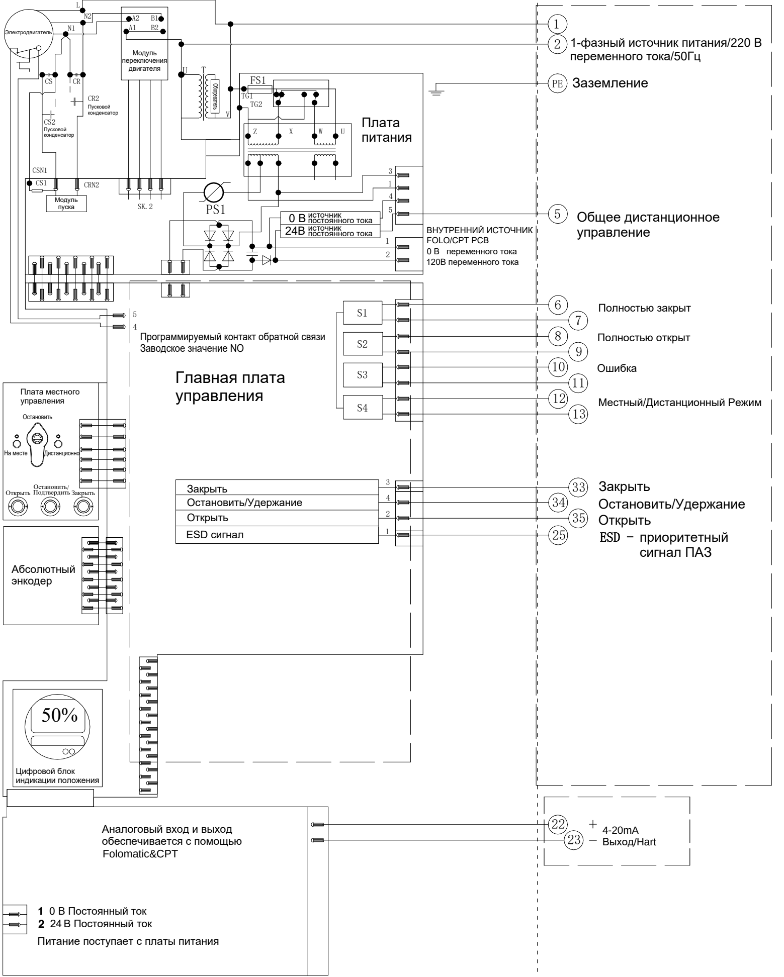
Электрическая схема №1-220-24-4-HR-3 Серия VAD
