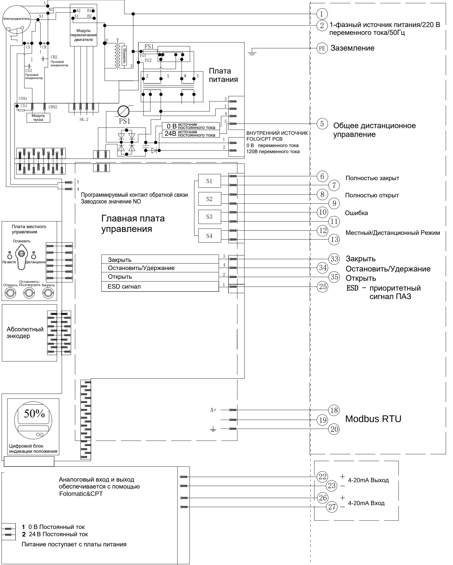
Электрическая схема №1-220-24-4-MR-1 Серия VAD
