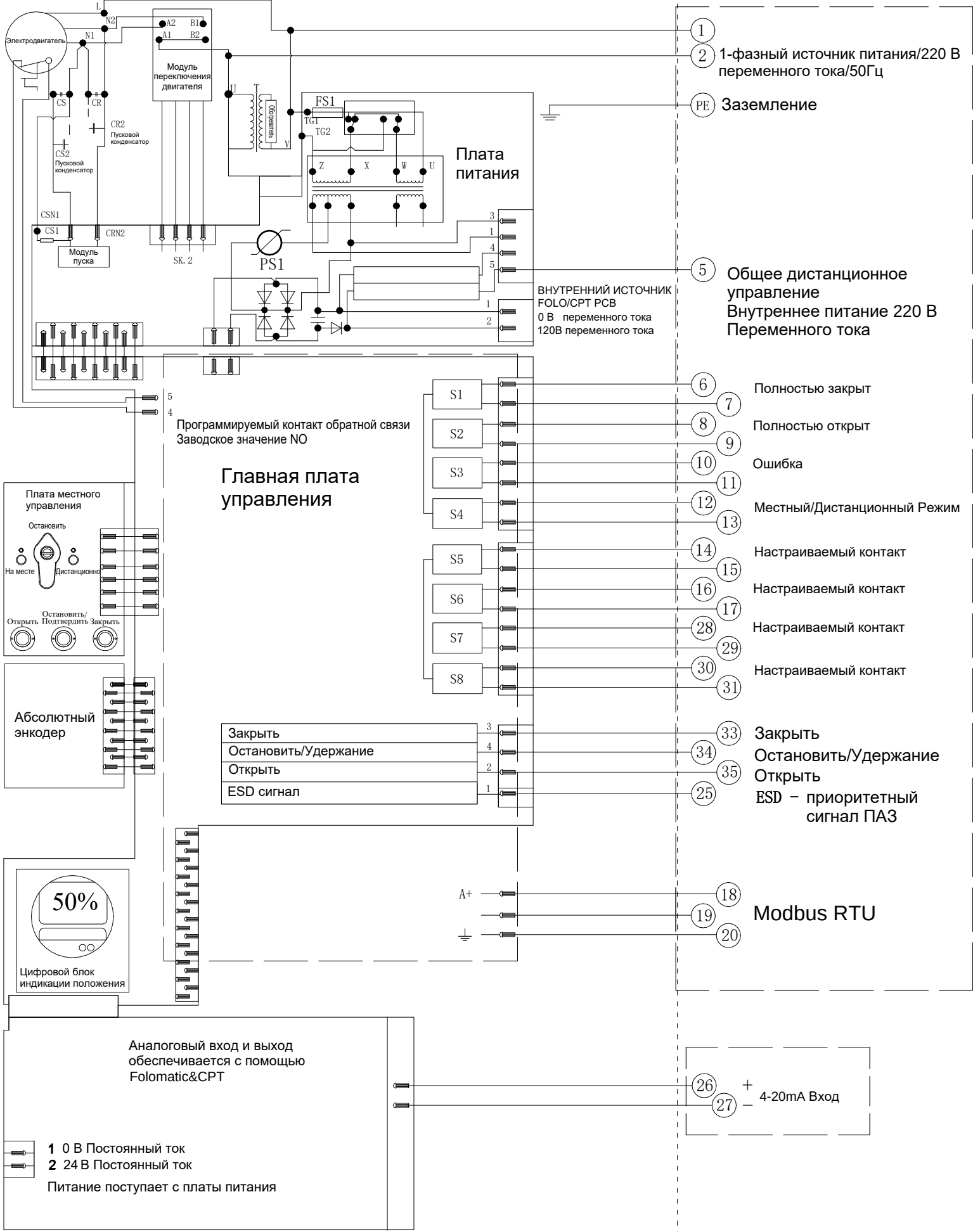
Электрическая схема №1-220-24-8-MR-2 Серия VAD
