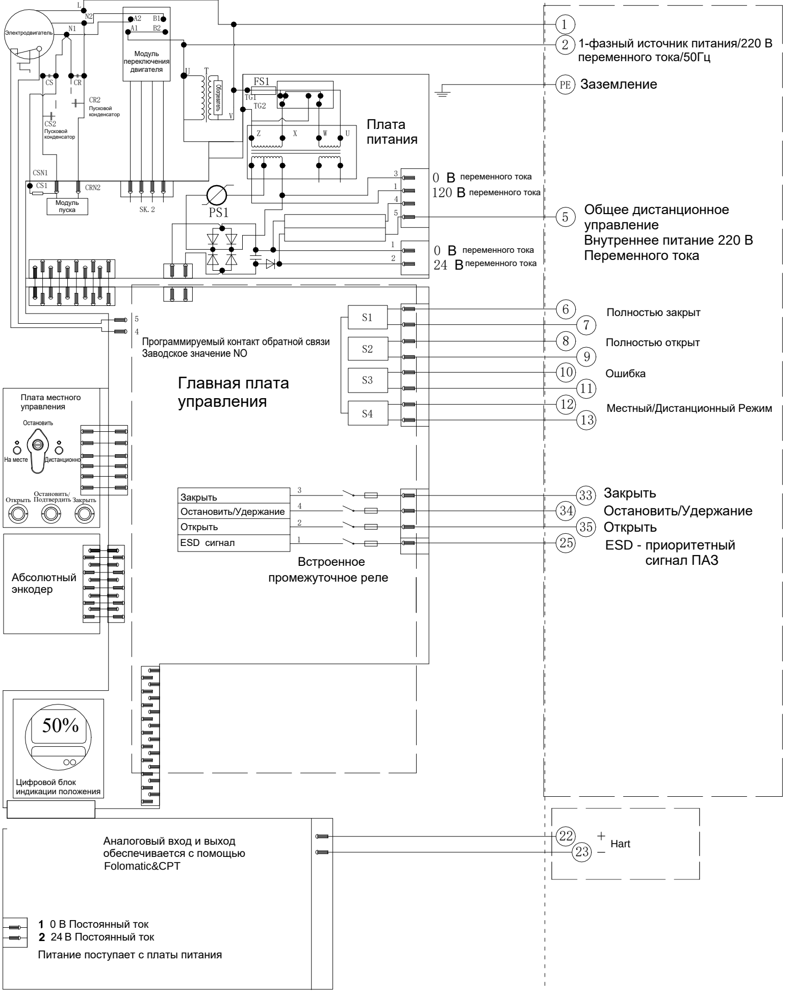
Электрическая схема №1-220-220-4-HR- 0 Серия VAD
