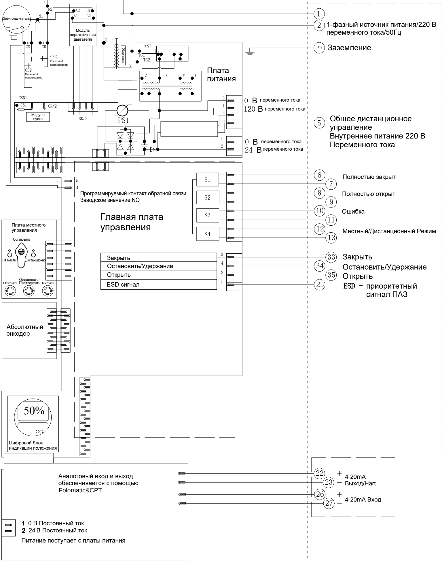
Электрическая схема №1-220-220-4-HR- 1 Серия VAD
